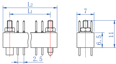
插座 XFC-ZSY:
